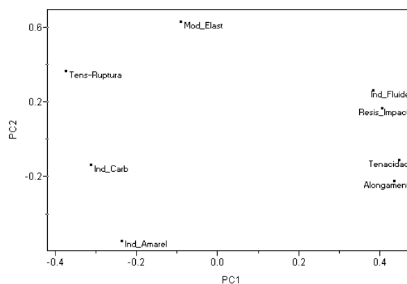
Figura 11: Loadings da propriedades do ABS.
