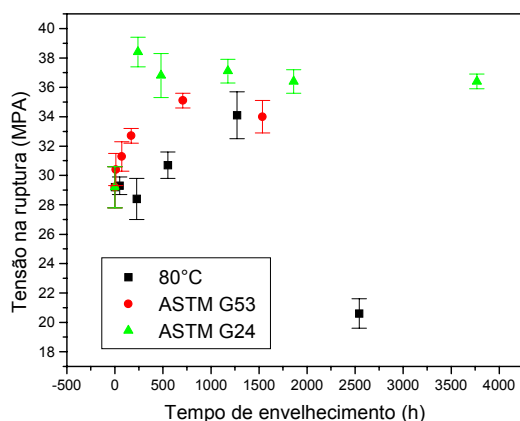
Figura 1: Tensão na ruptura para o ABS em função do tempo de envelhecimento e da técnica utilizada.
