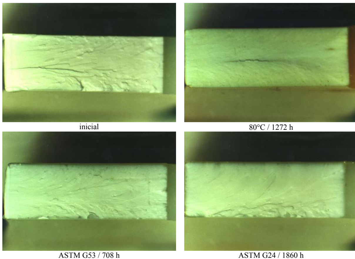
Figura 9: Fraturas obtidas nos ensaios de impacto do ABS (aumento de 7 vezes).
