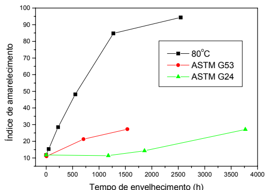
Figura 6: Índice de amarelecimento para o ABS.
