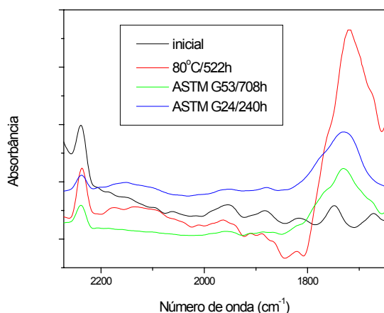
Figura 7: Espectros na região de infravermelho nas regiões de absorção CN ( 2236\text{ cm}^{-1} ) e de carbonilas ( 1746\text{ cm}^{-1} ).
