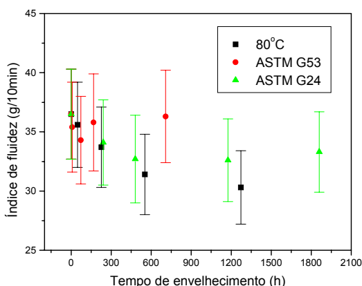
Figura 5: Índice de fluidez para o ABS.
