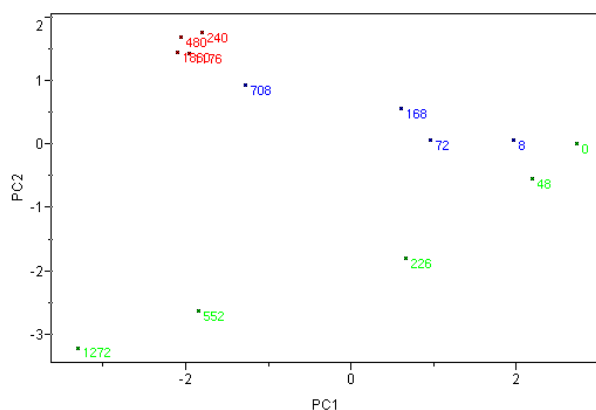
Figura 10: Scores em relação ao método de envelhecimento para o ABS (verde: térmico, azul: ASTM G53, vermelho: ASTM G24).
